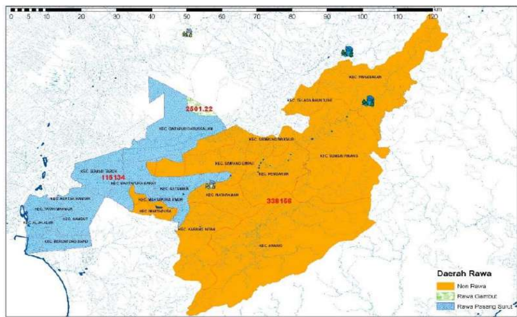
Gambar 2. 7. Daerah Aliran Sungai (DAS) di Kabupaten Banjar
