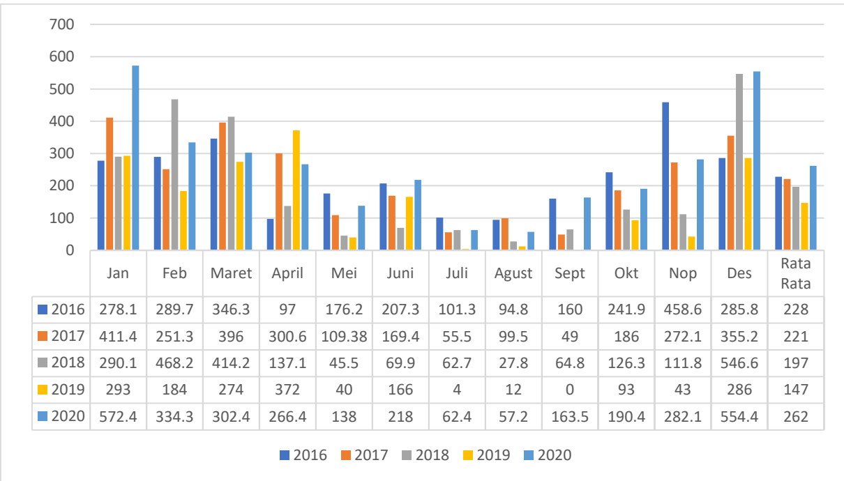
Gambar 2. 8. Gambar Curah Hujan di Kabupaten Banjar Tahun 2016 - 2020
